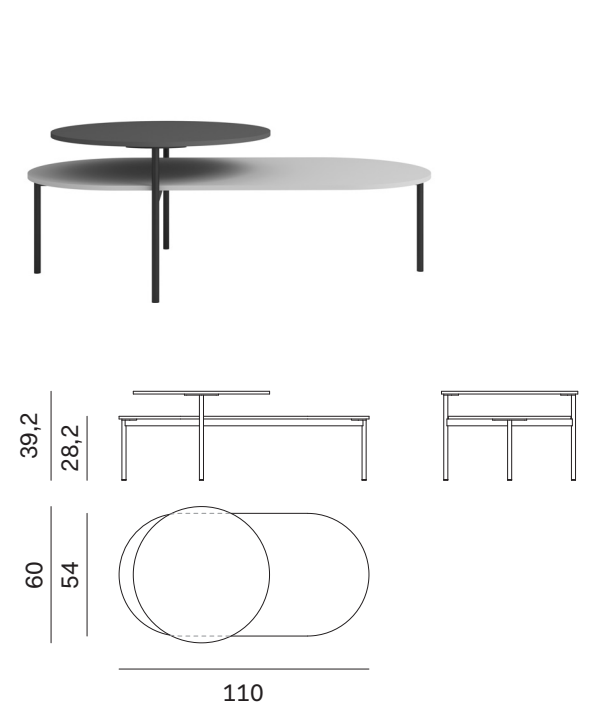
Tavolino L. 110 110cm-wide coffee table
